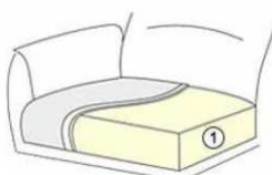
HR ① Schaum HR 38kg/m³
