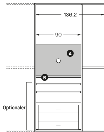
Schrankabteil B. 136,2 für TV-Gerät
