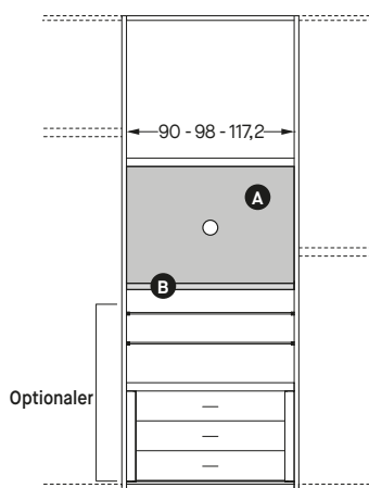
Schrankabteil B. 90 - 98 - 117,2 für TV-Gerät
